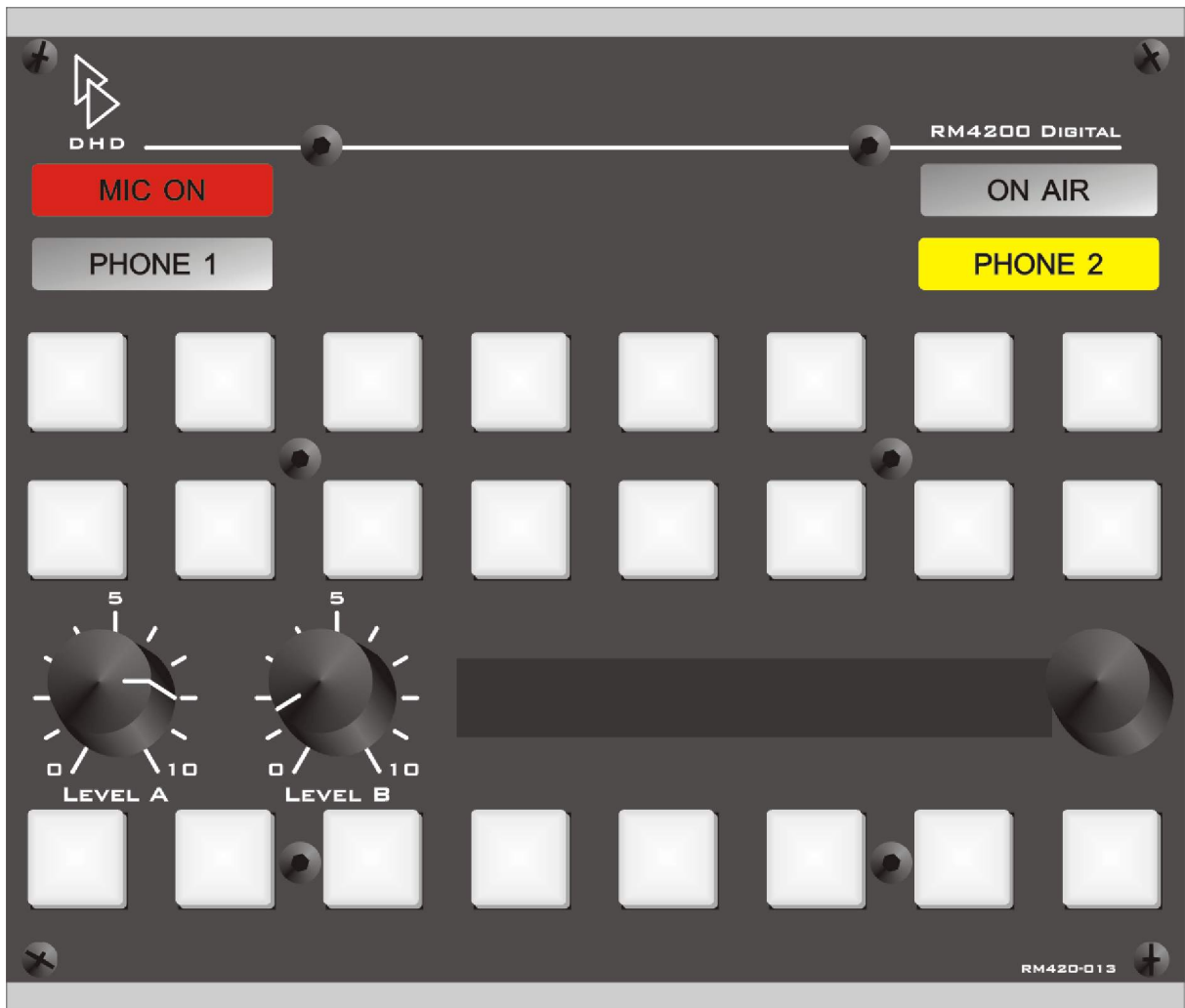
RM420-013L print layout for DIN A4
