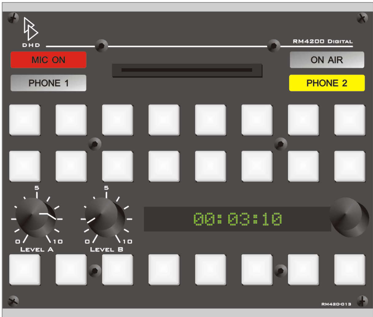
RM420-013 print layout for DIN A4
