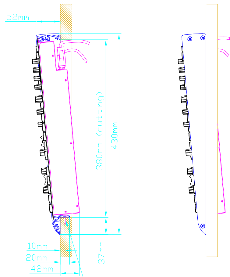
Cut A-A
